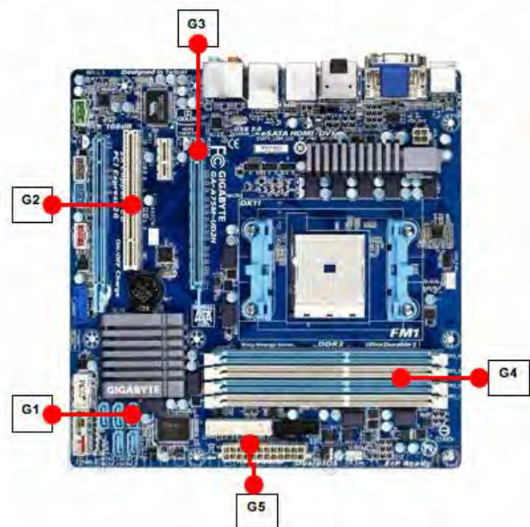
Placa mãe Gigabyte – GA–A75M-UD2H
