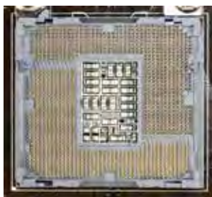
Soquete LGA1156
