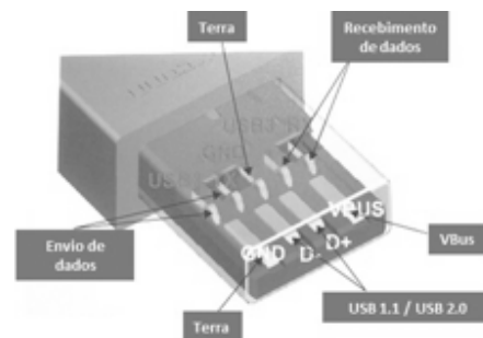
Detalhes do conector USB
